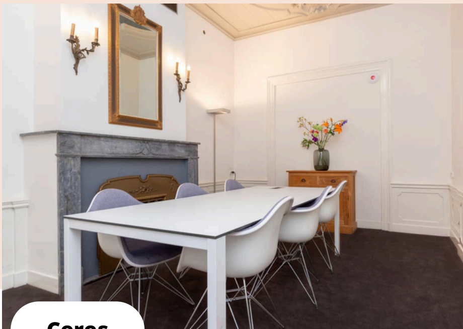
Ceres
