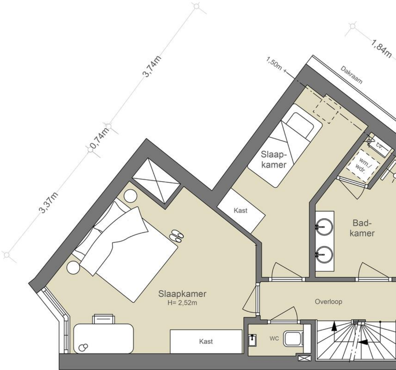
3 e VERDIEPING
